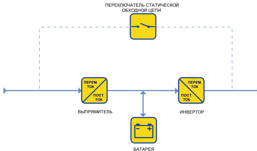
Рис. 4 – Оперативные (on-line) ИБП с двойным преобразованием
