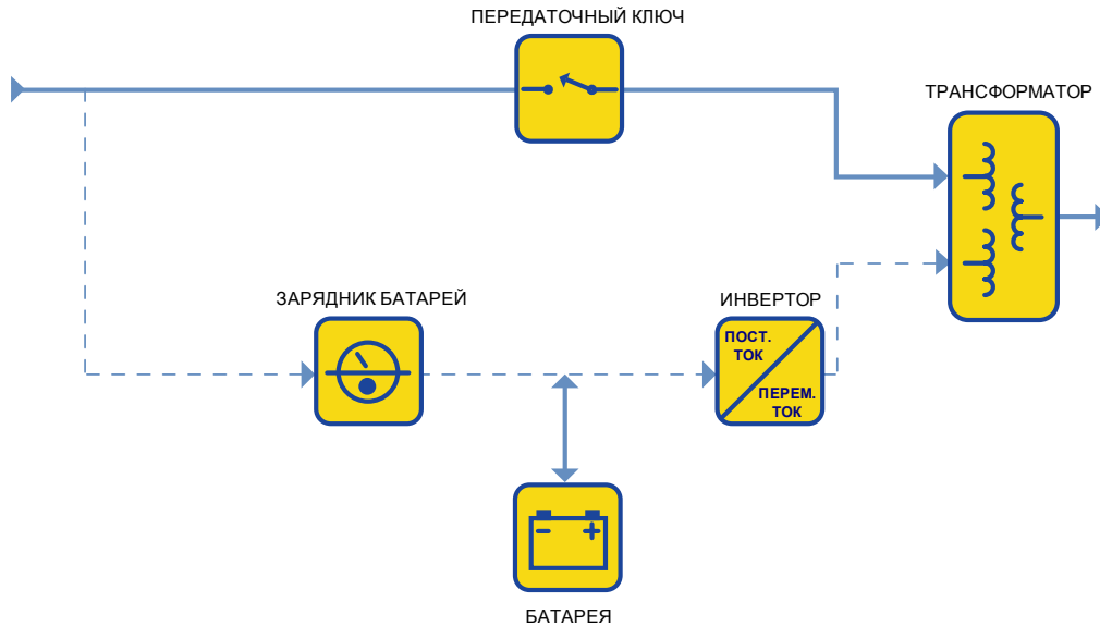
Рис. 3 - Резервные ИБП с ферромагнитами
