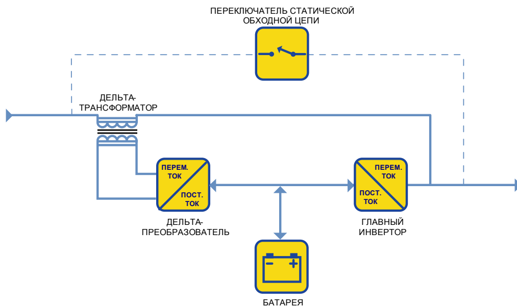
Рис. 5 - Оперативные ИБП с дельта-преобразованием
