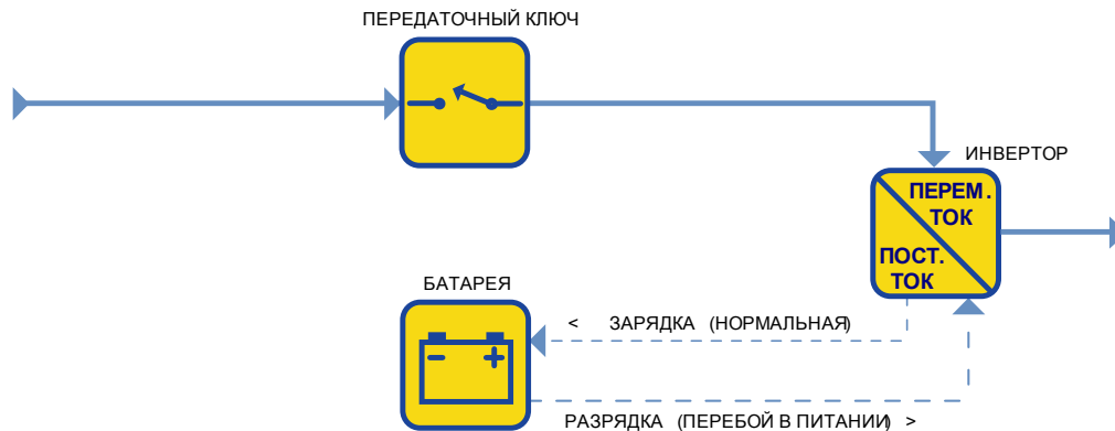
Рис. 2 - Линейно-интерактивные ИБП
