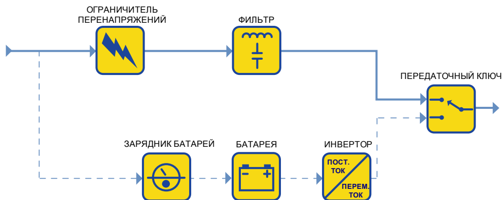
Рис. 1 - Резервные ИБП
