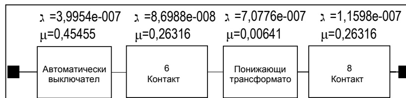
Рис. 16. Детали трансформатора
